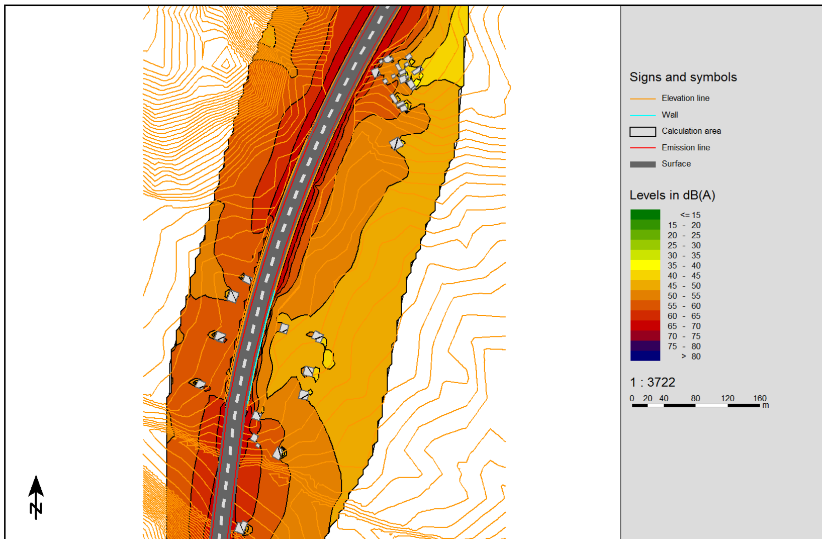
Слика 18 Мапа на бучавата ( L_n ) меѓу стационажите 11+243 и 12+051 без заштитни бариери
