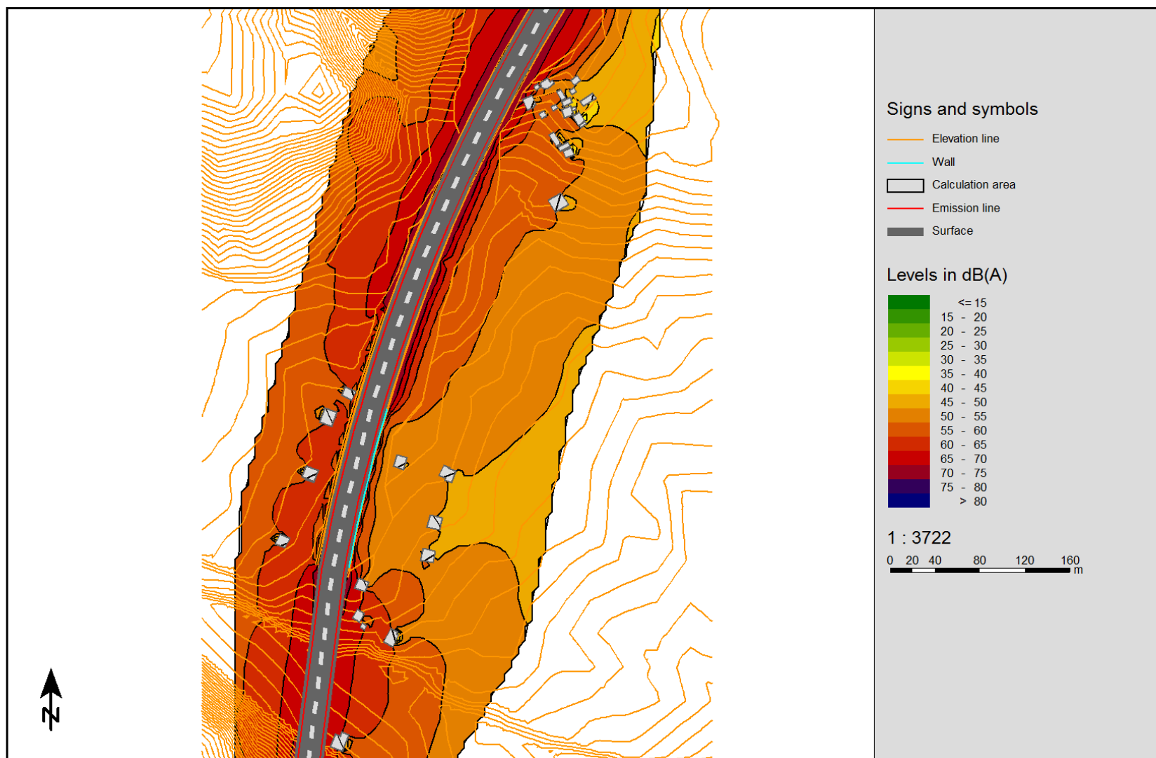
Слика 16 Мапа на бучавата (Le) меѓу стациоњите 11+243 и 12+051 без заштитни бариери
