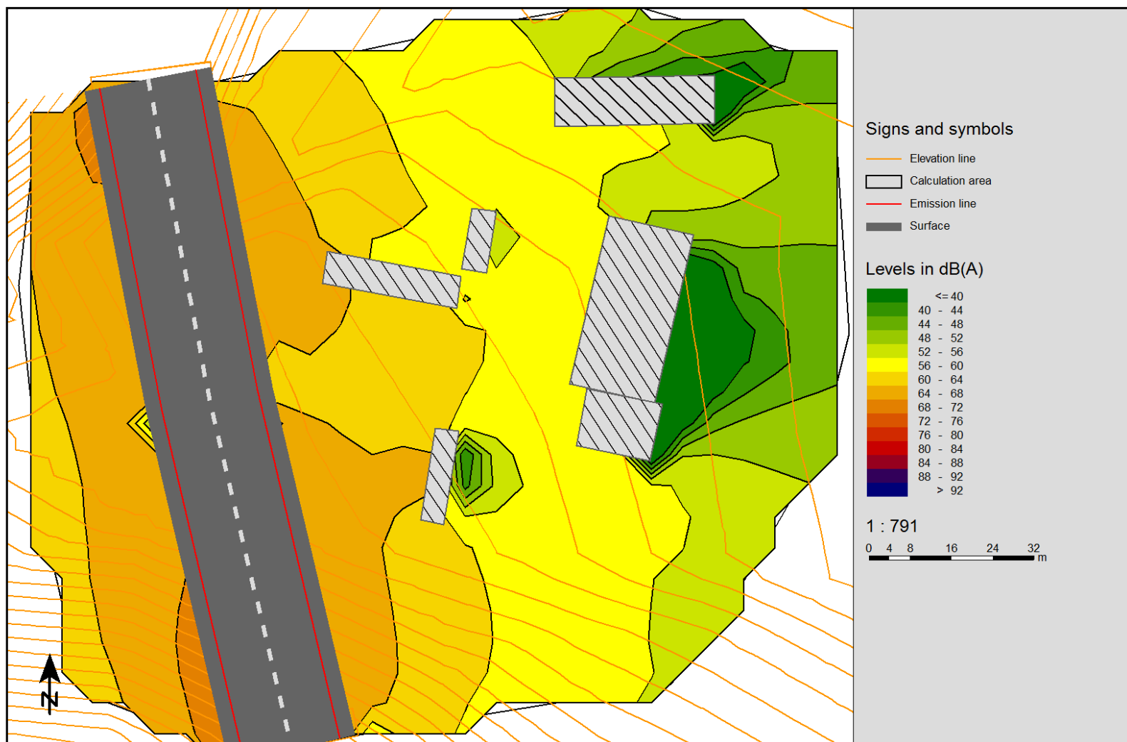
Слика 26 Мапа на бучавата ( L_n ) меѓу стационите 11+243 и 12+051 без заштитни бариери
