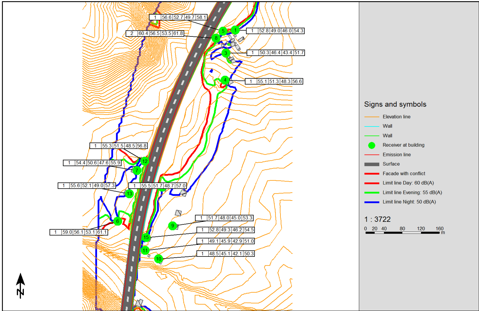
Слика 13 Бучава на поединечни точки долж трасата меѓу стационите 2+780 и 2+940 со заштитни бариери
