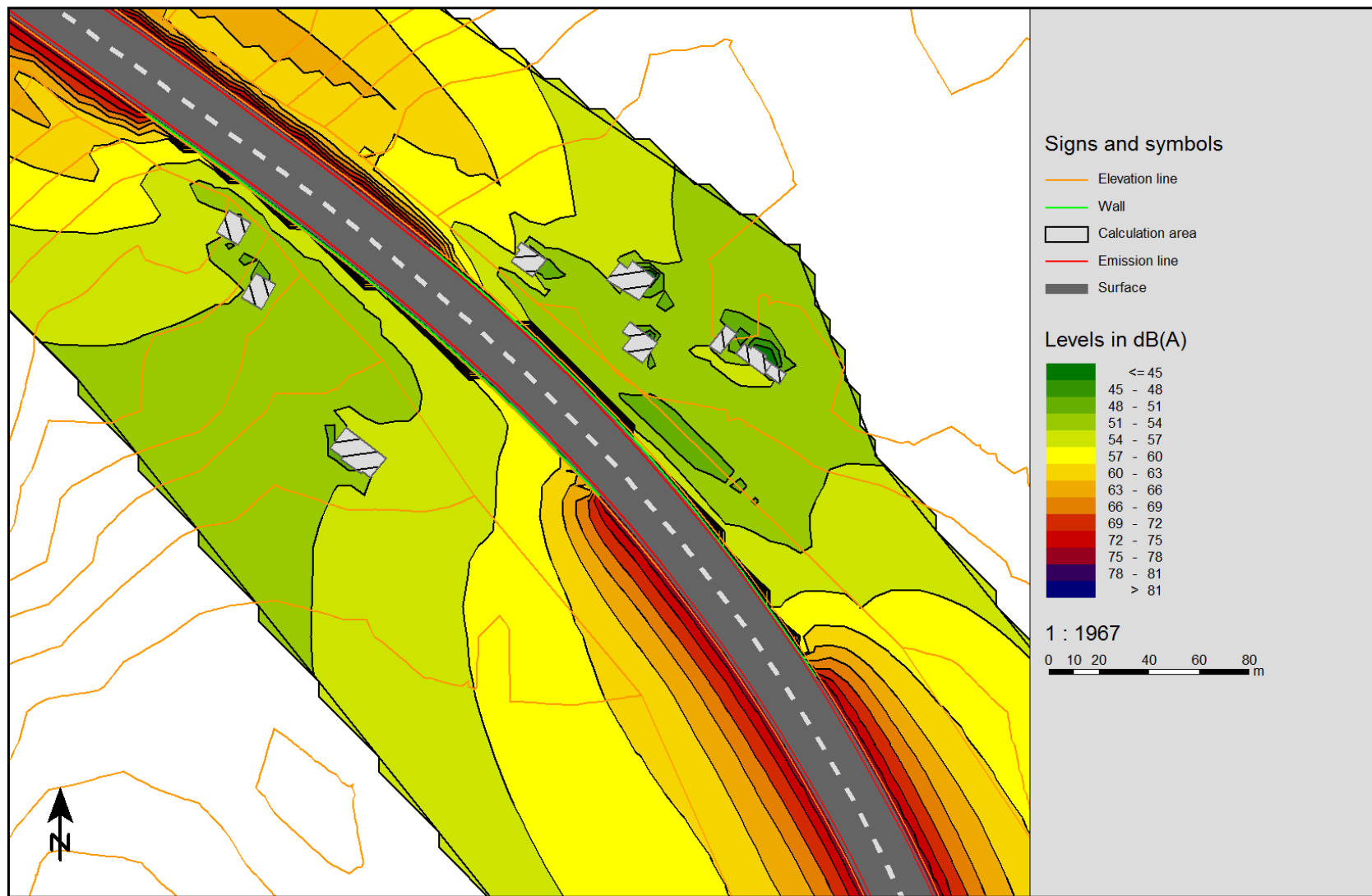
Слика 9 Слика 6 Мапа на бучавата (Lv) меѓу стациоанжите 2+780 и 2+940 со заштитни бариери
