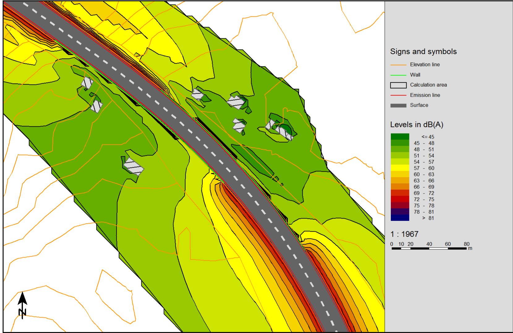
Слика 11 Слика 6 Мапа на бучавата (Ln) меѓу стациоажите 2+780 и 2+940 со заштитни бариери
