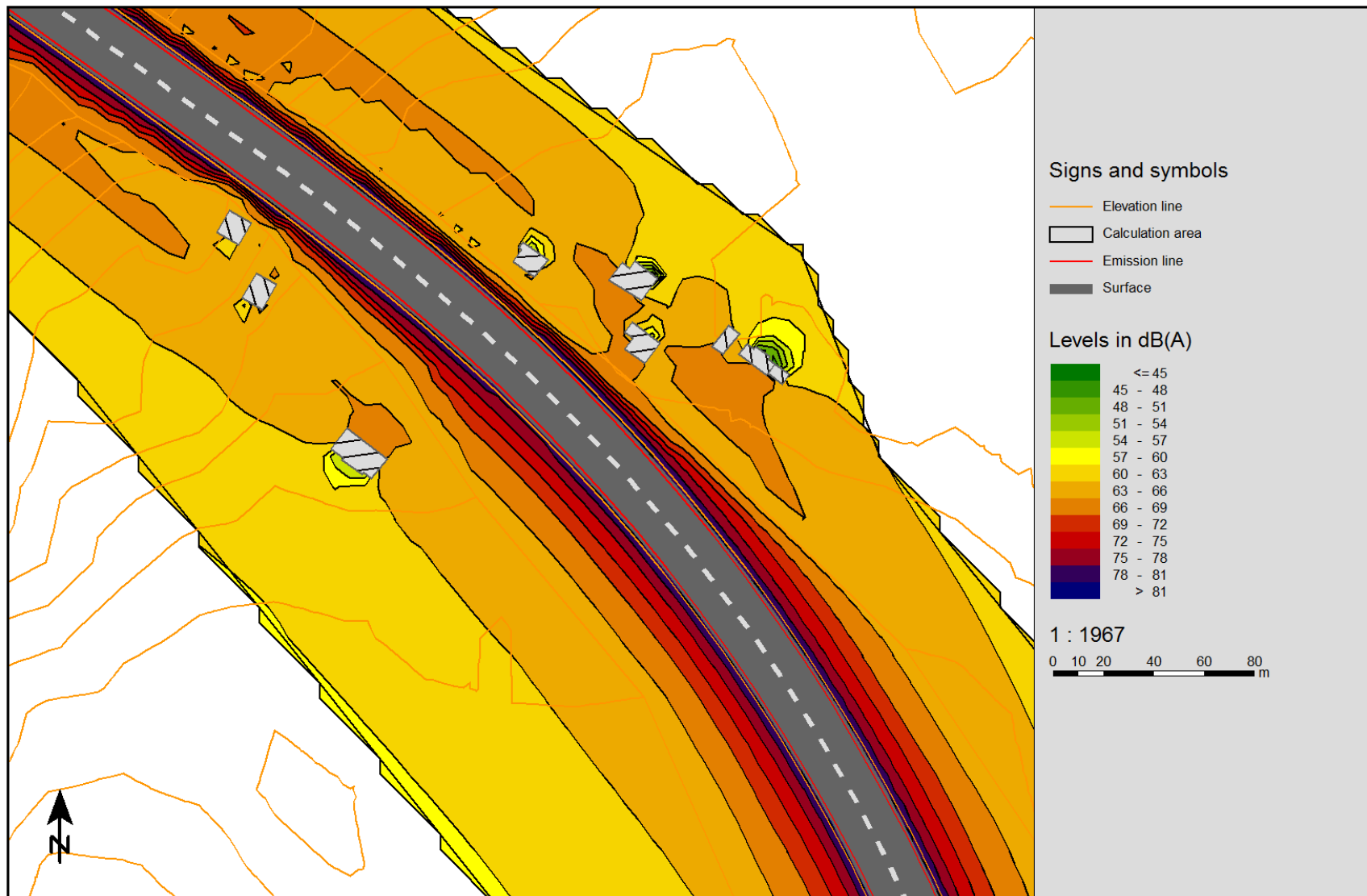
Слика 6 Мапа на бучавата (Ld) меѓу стациоите 2+780 и 2+940 без заштитни бариери
