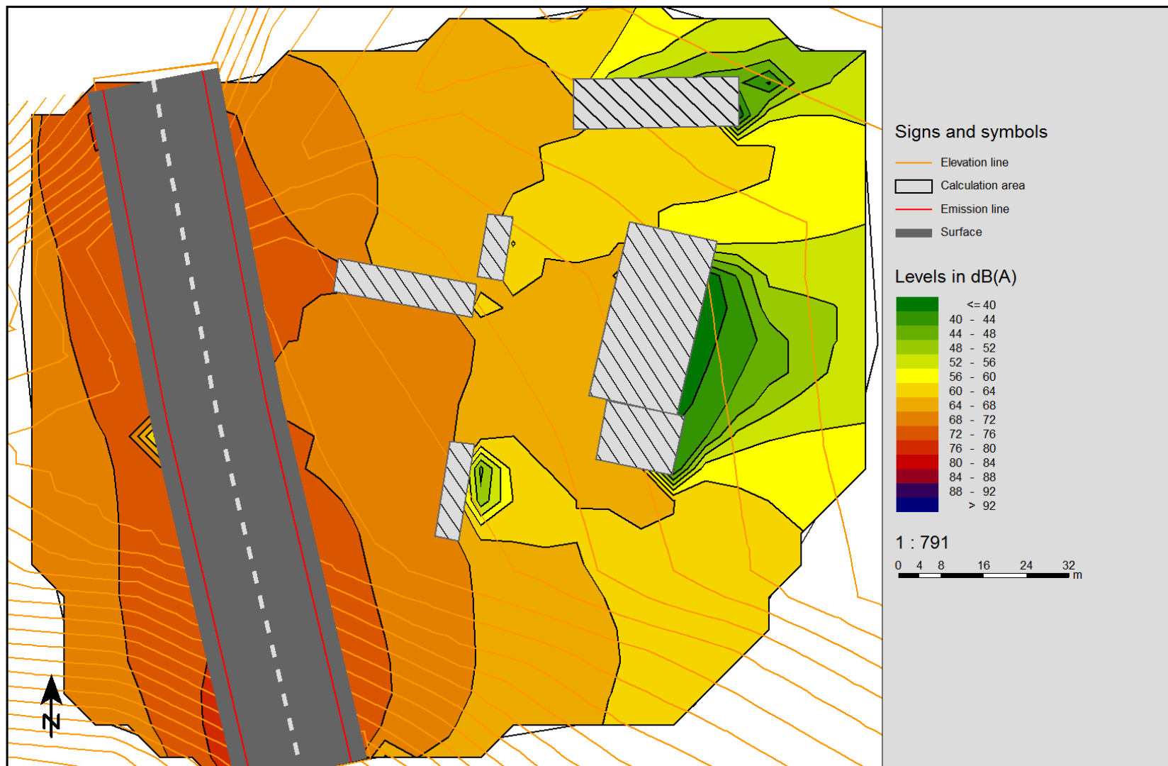
Слика 22 Мапа на бучавата (Ld) меѓу стационите 12+412 и 12+542 без заштитни бариери
