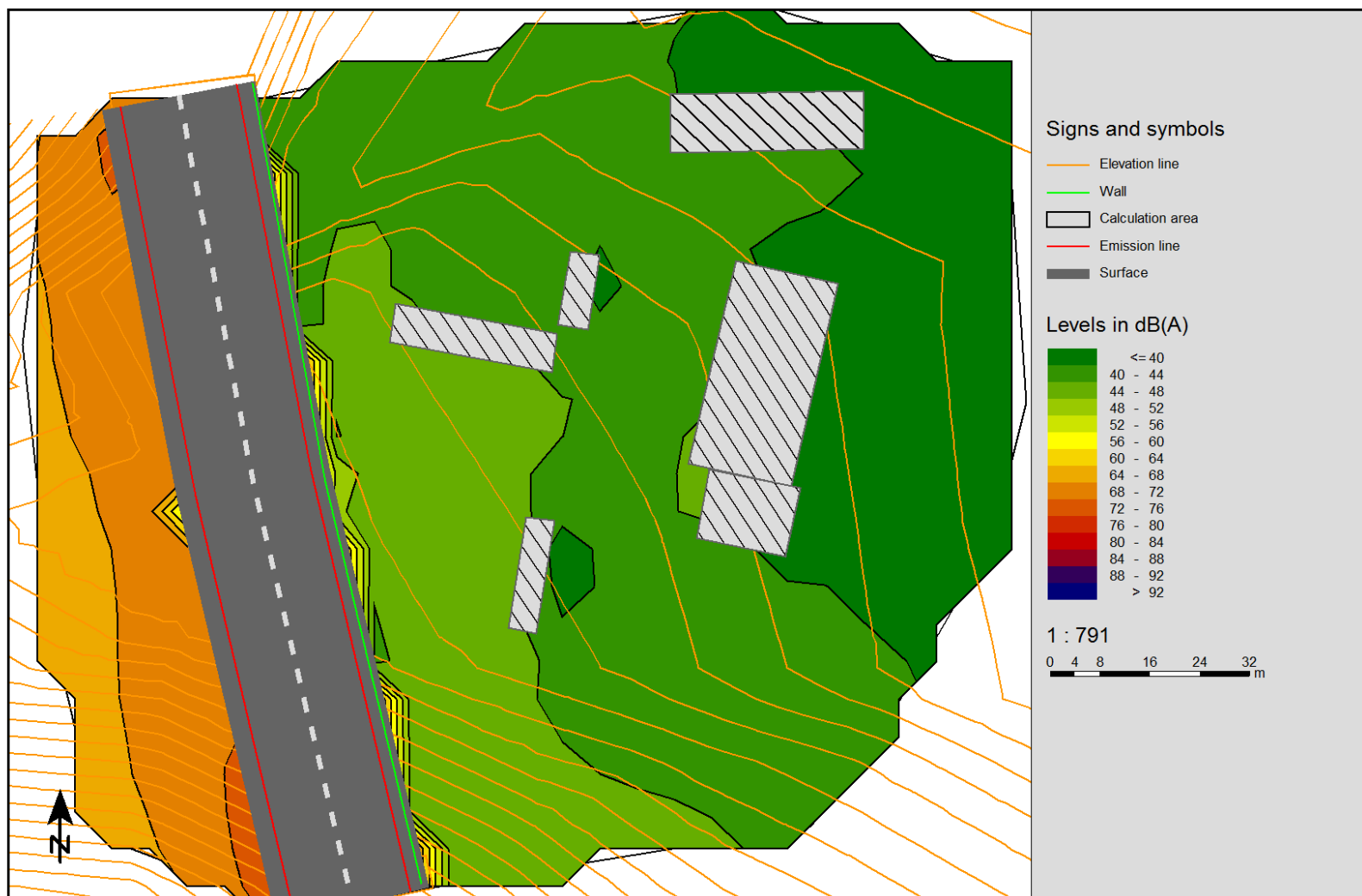
Слика 25 Мапа на бучавата (Lv) меѓу стационите 11+243 и 12+051 со заштитни бариери
