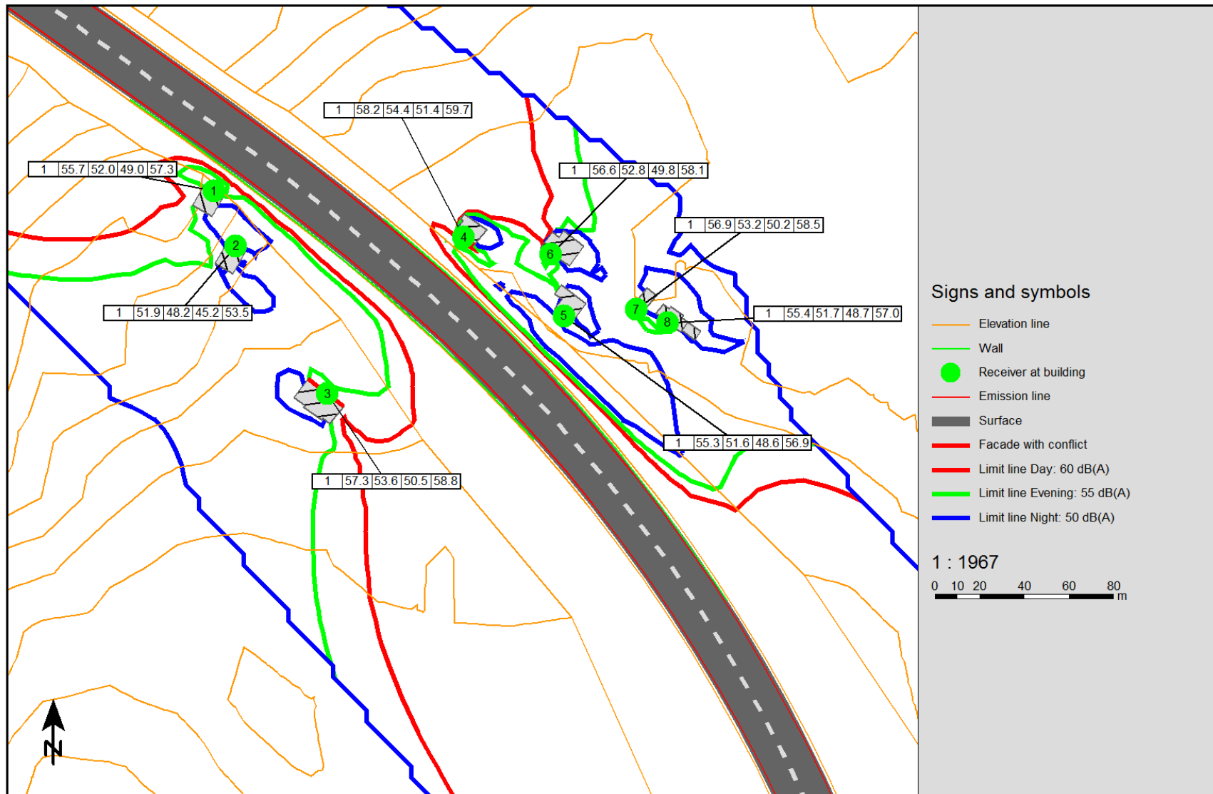
Слика 5 Бучава на поединечни точки долж трасата меѓу стациоњите 2+780 и 2+940 со заштитни бариери
