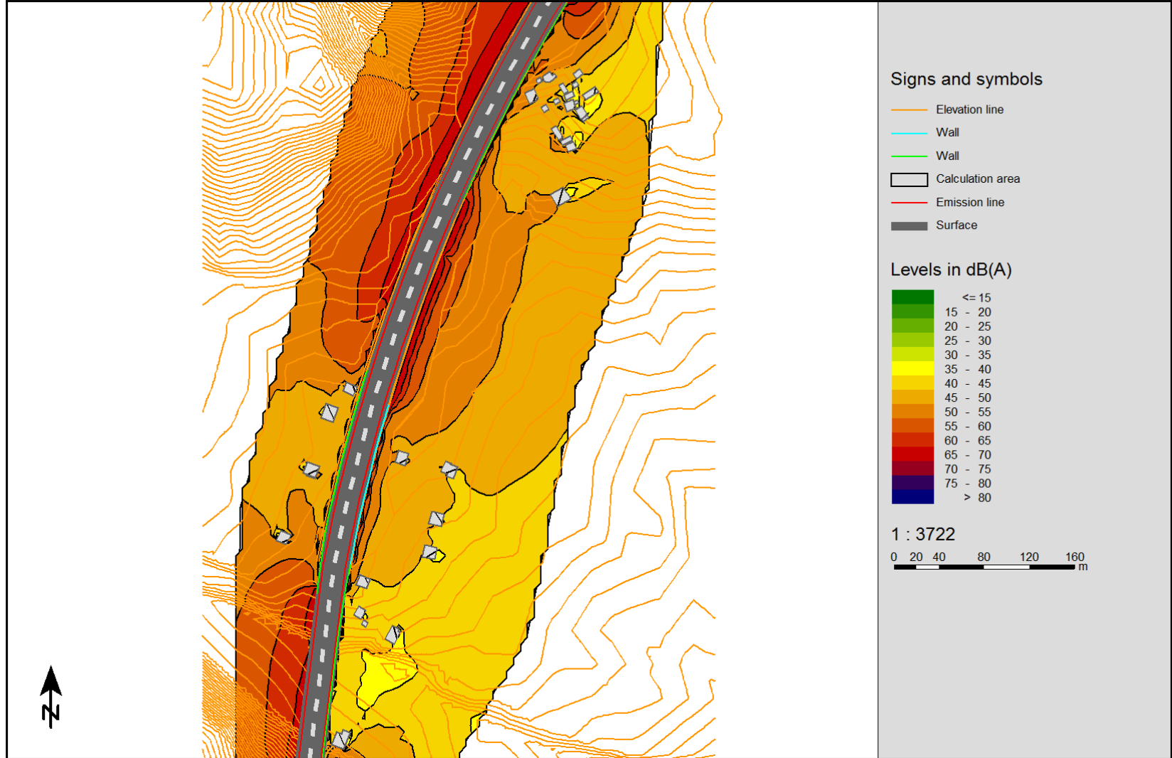
Слика 19 Мапа на бучавата (Ln) меѓу стациоите 11+243 и 12+051 со заштитни бариери
