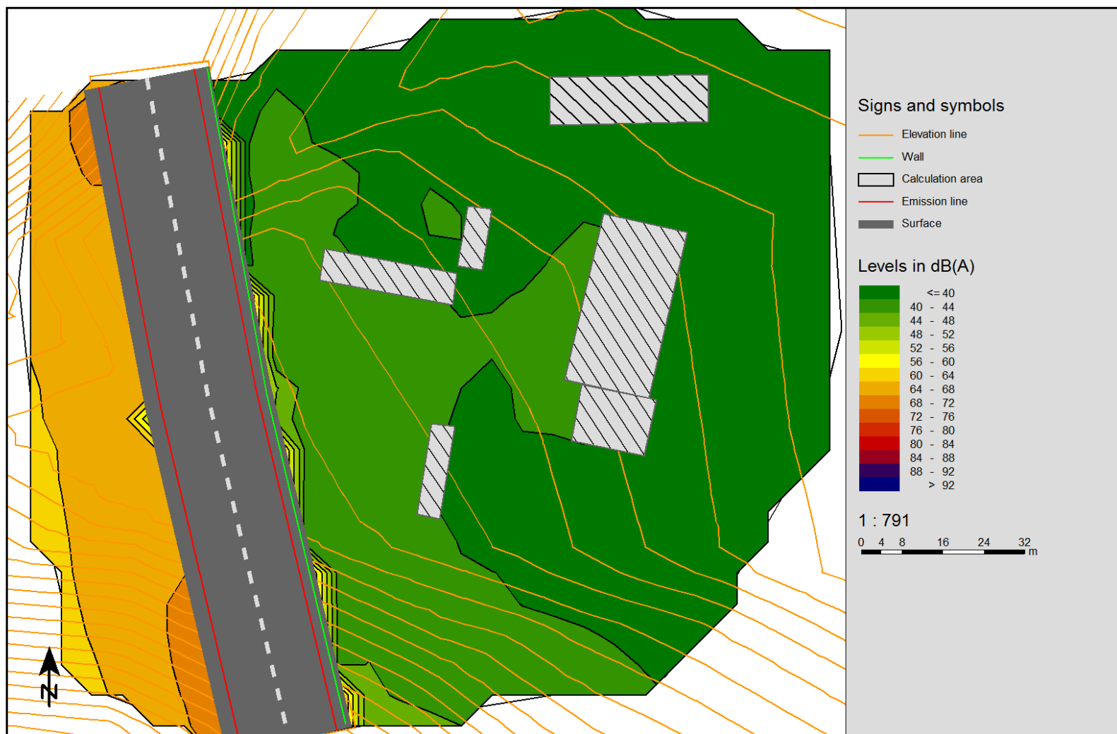
Слика 27 Мапа на бучавата (Ln) меѓу стационите 11+243 и 12+051 со заштитни бариери
