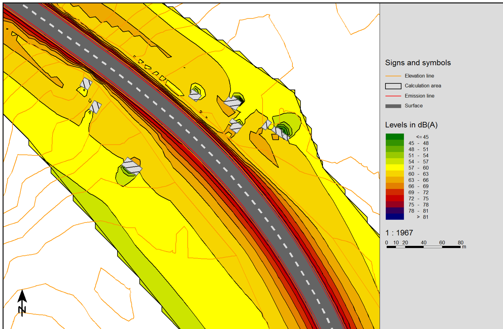
Слика 8 Слика 6 Мапа на бучавата (Lv) меѓу стационажите 2+780 и 2+940 без заштитни бариери
