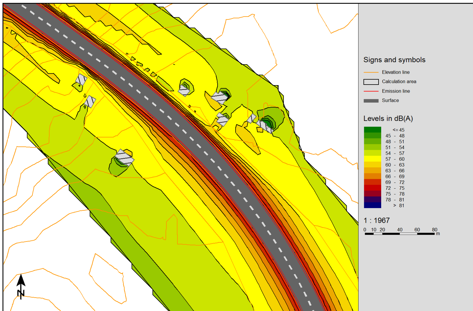
Слика 10 Слика 6 Мапа на бучавата (Ln) меѓу стациоаните 2+780 и 2+940 без заштитни бариери
