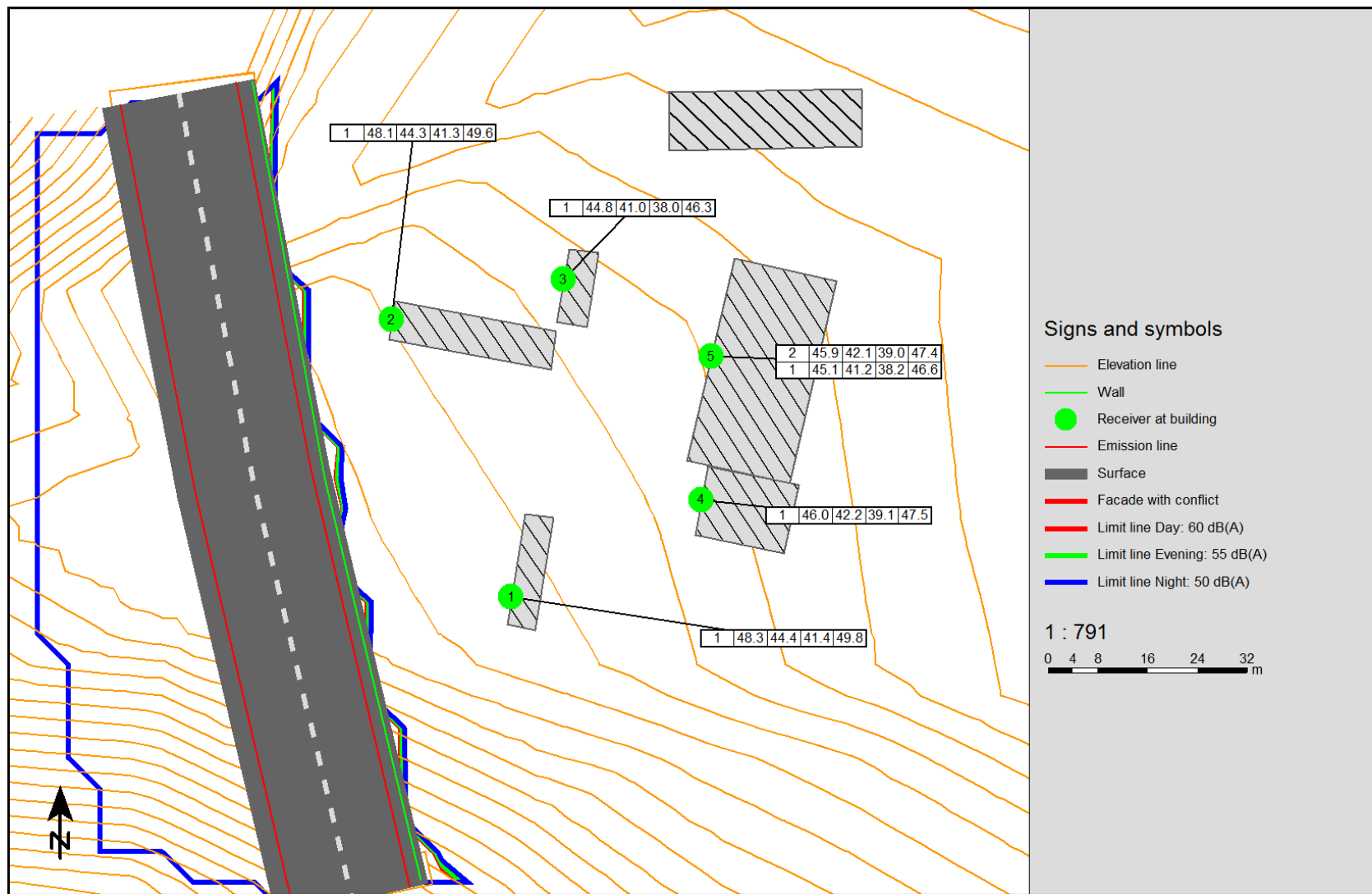
Слика 21 Резултати од пресметките (Sound Plan Essential) на бучавата кај осетливите рецептори меѓу стационите 12+412 и 12+542 со звучни бариери
