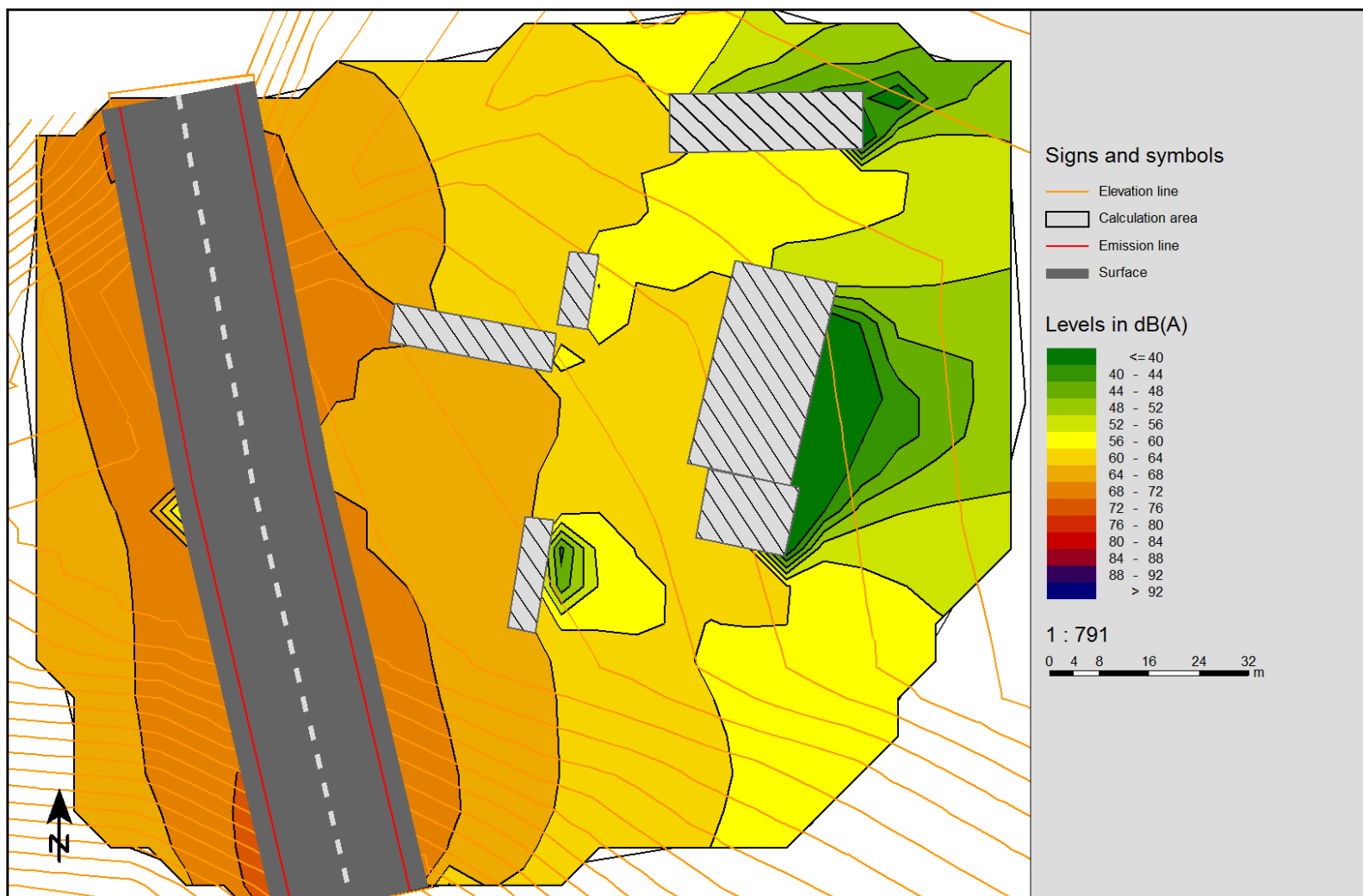
Слика 24 Мапа на бучавата (Lv) меѓу стациононите 11+243 и 12+051 без заштитни бариери
