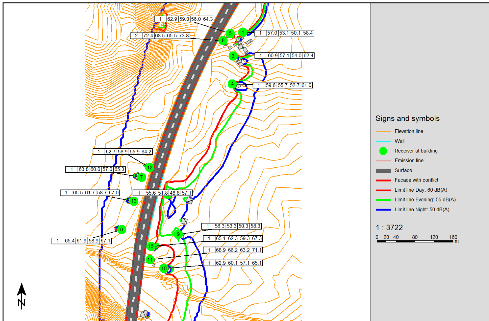
Слика 12 Бучава на поединечни точки долж трасата меѓу стационажите 11+243 и 12+051 без заштитни бариери
