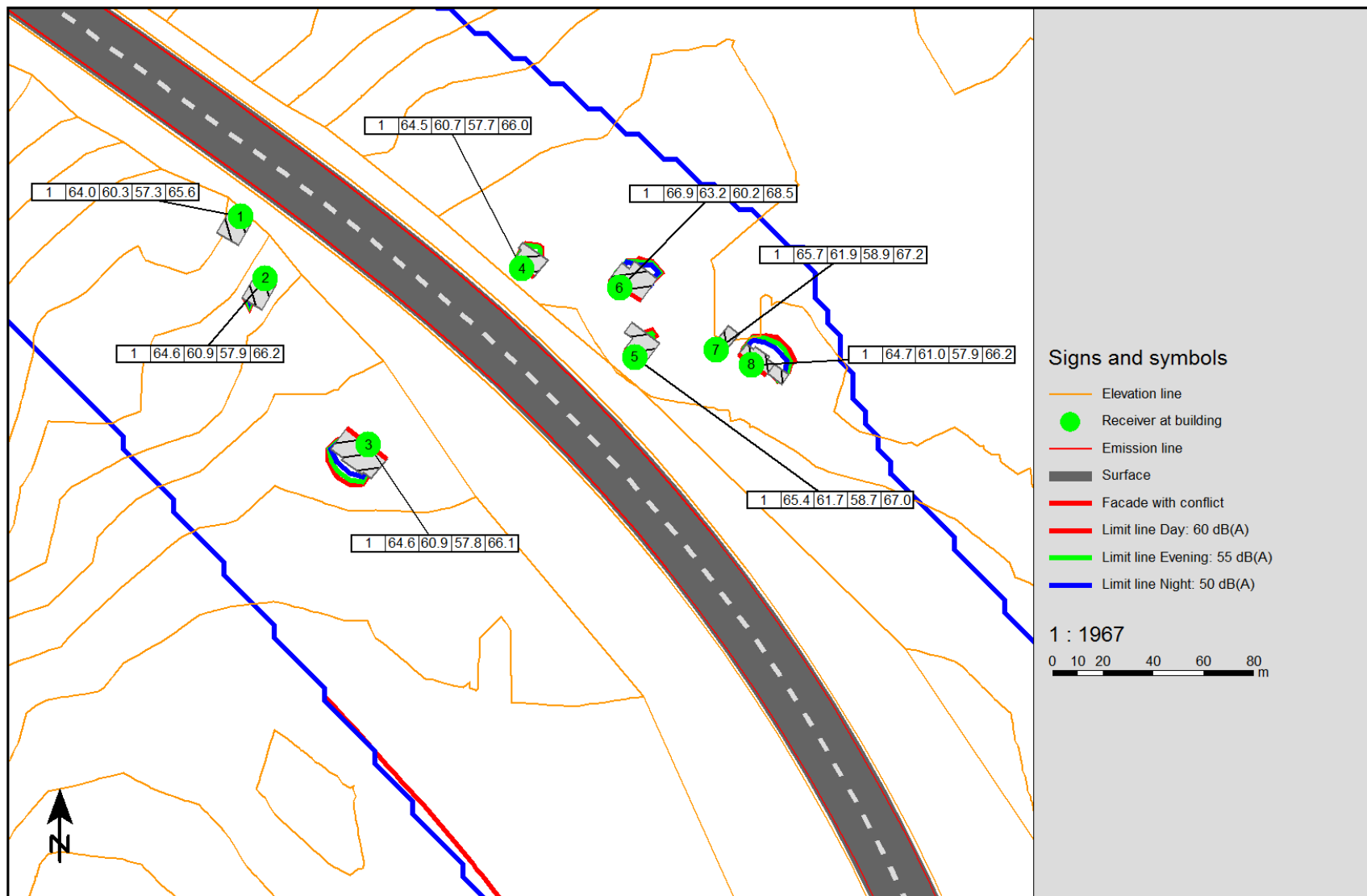
Слика 4 Бучава на поединечни точки долж трасата меѓу стациоажите 2+780 и 2+940 без заштитни бариери
