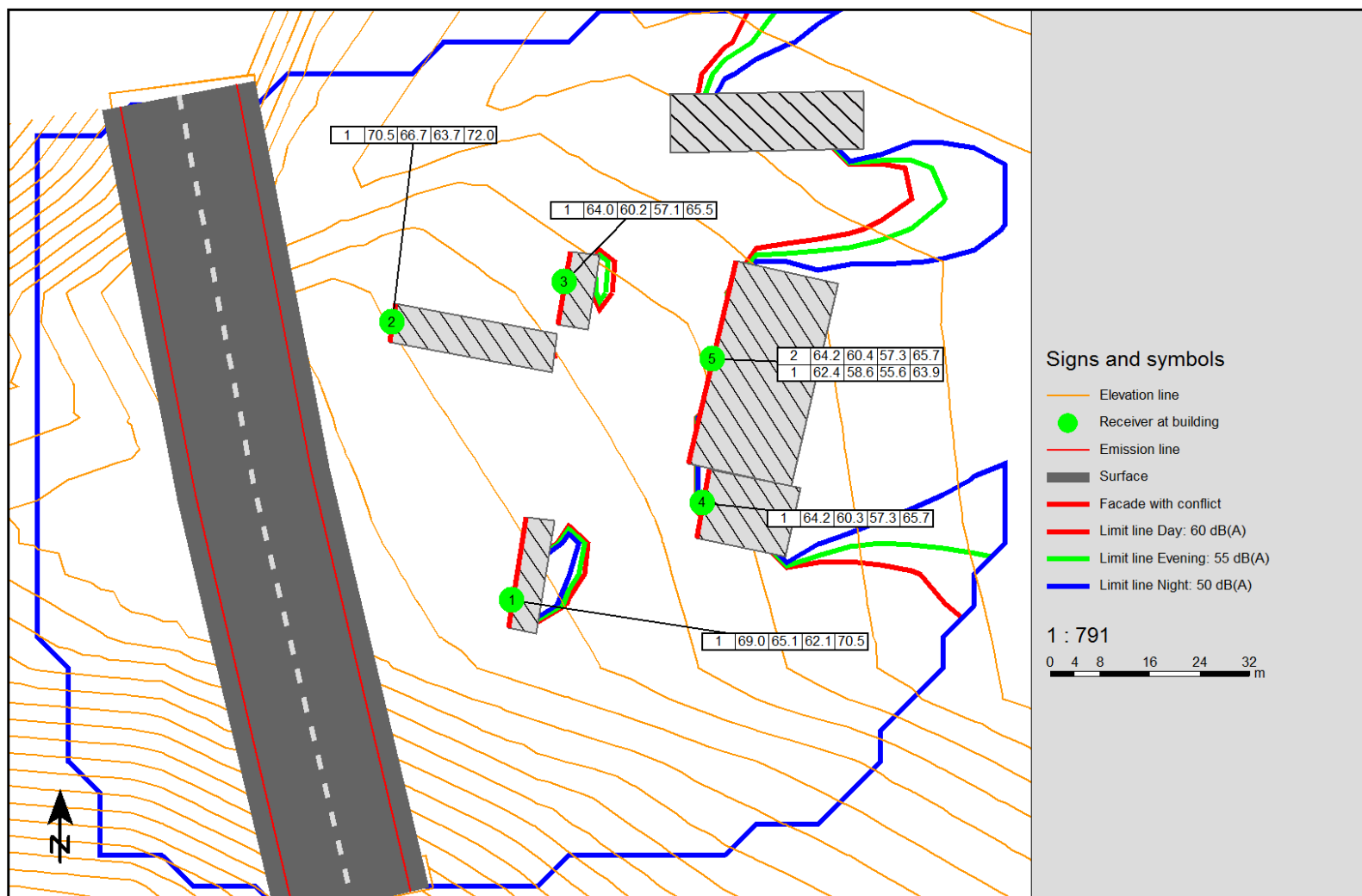
Слика 20 Резултати од пресметките (Sound Plan Essential) на бучавата кај осетливите рецептори меѓу стациоаните 12+412 и 12+542 без звуќни бариери
