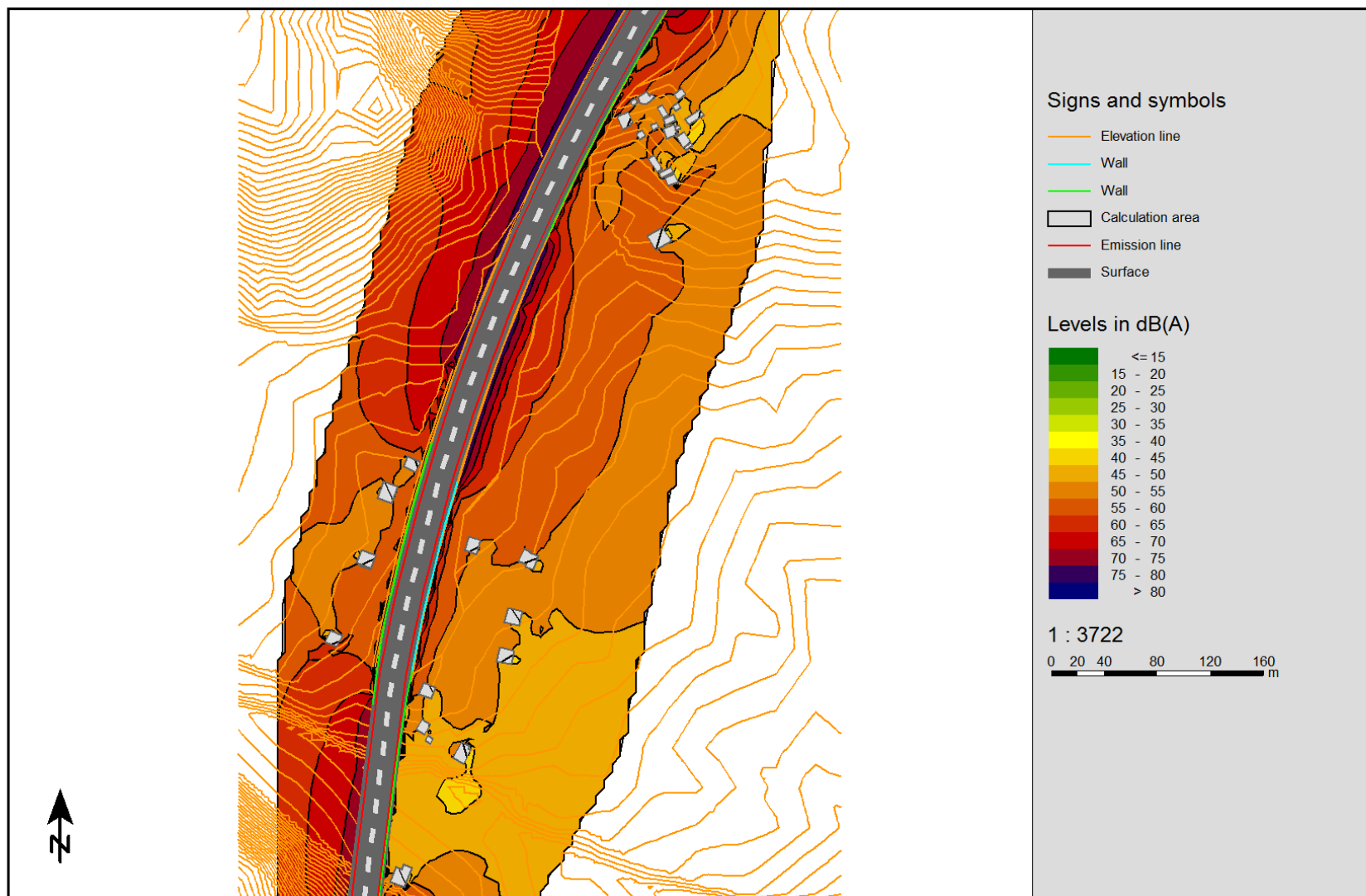
Слика 15 Мапа на бучавата (Ld) меѓу стационачите 11+243 и 12+051 со заштитни бариери
