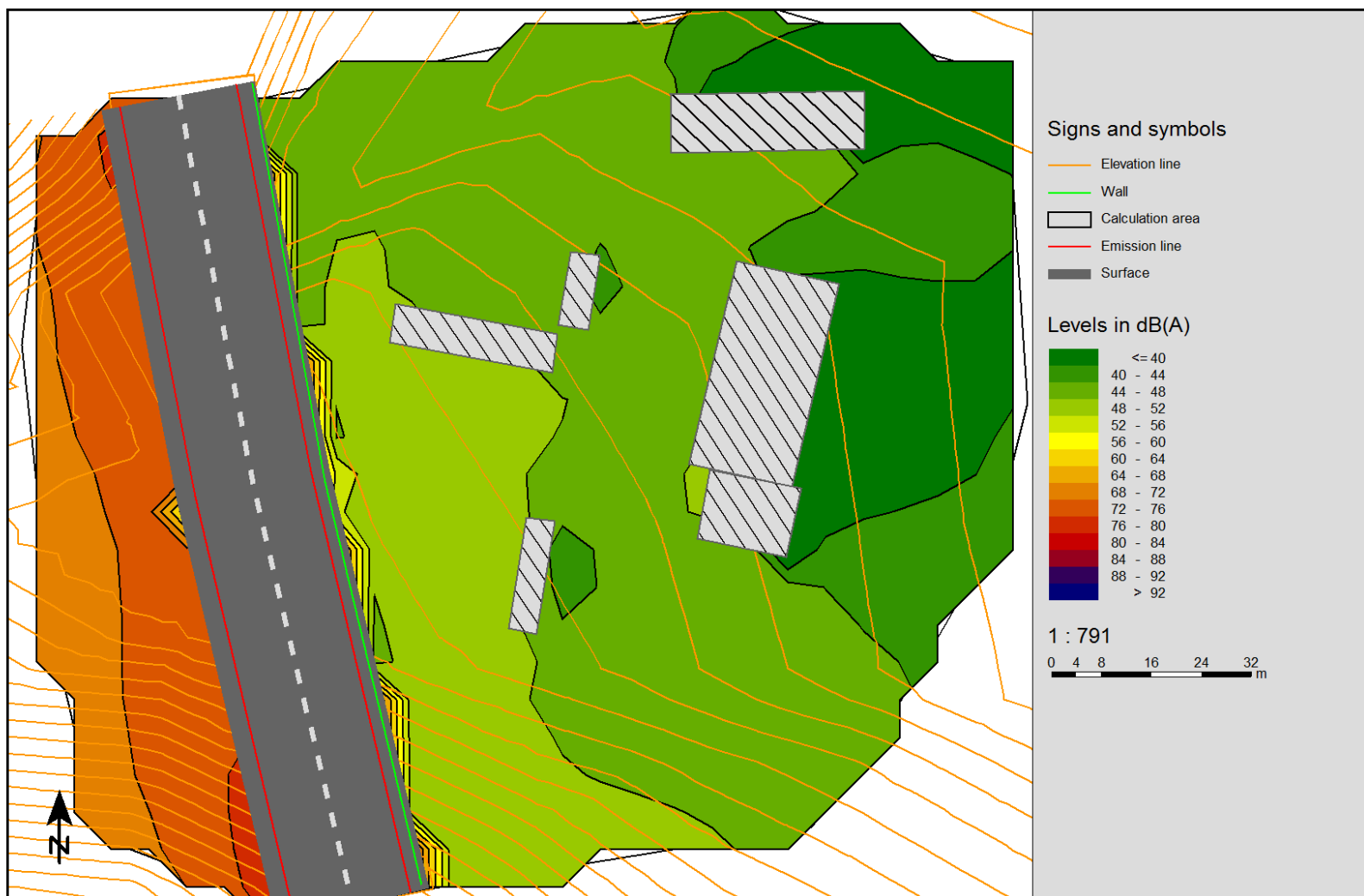
Слика 23 Мапа на бучавата (Ld) меѓу стационите 11+243 и 12+051 со заштитни бариери
