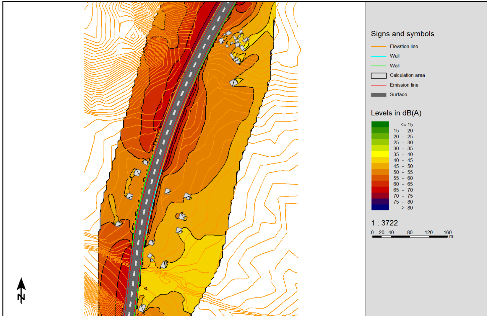
Слика 17 Мапа на бучавата (Le) меѓу стациоњите 11+243 и 12+051 со заштитни бариери
