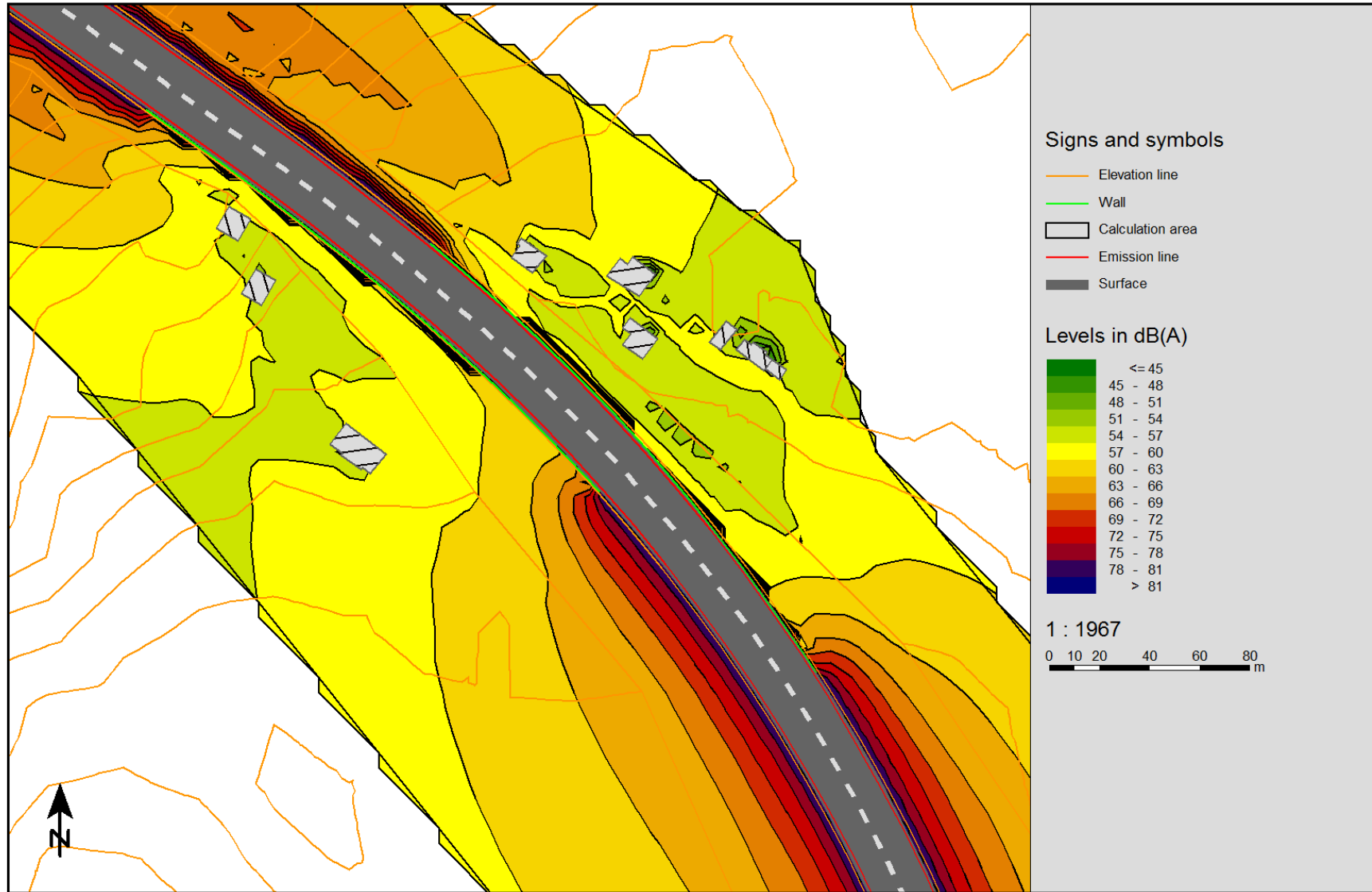
Слика 7 Слика 6 Мапа на бучавата (Ld) меѓу стациоаните 2+780 и 2+940 со заштитни бариери
