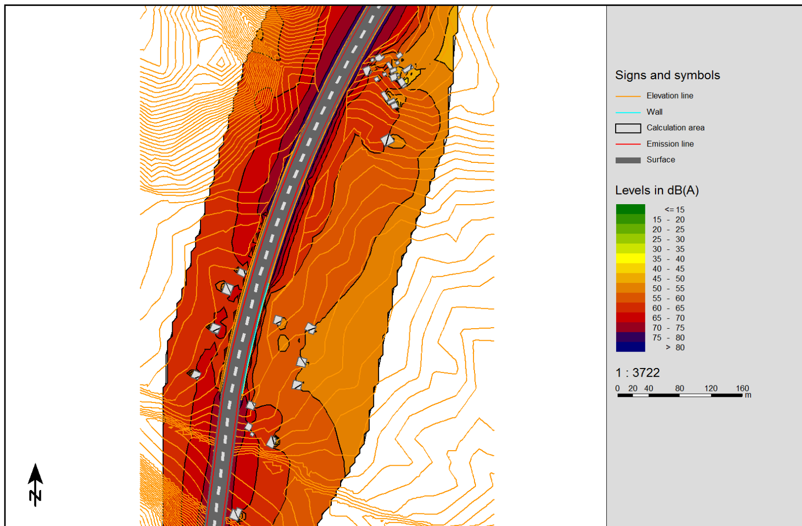
Слика 14 Мапа на бучавата ( L_d ) меѓу стациоажите 11+243 и 12+051 без заштитни бариери
