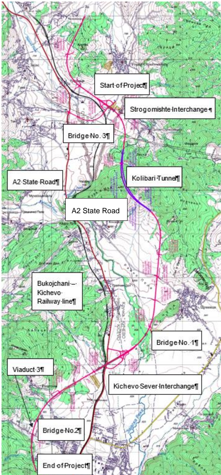
Figura 4-1–Shtrirja e Projektit
