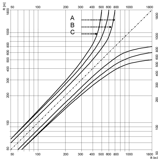
Слика 29. Односи на редоследот на радиусите на лаците
