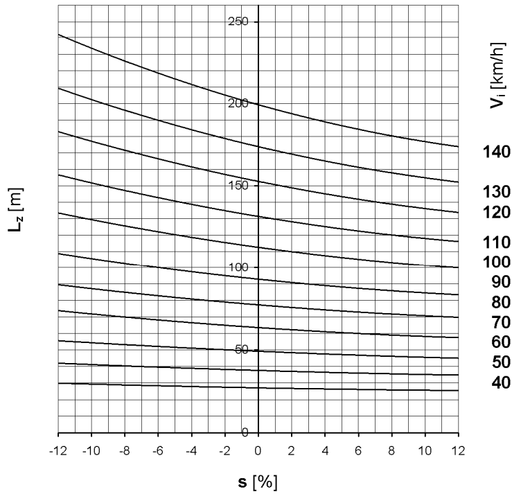
Слика 21. Скратена прегледност за застанување ( f_{T 50 \%} )
