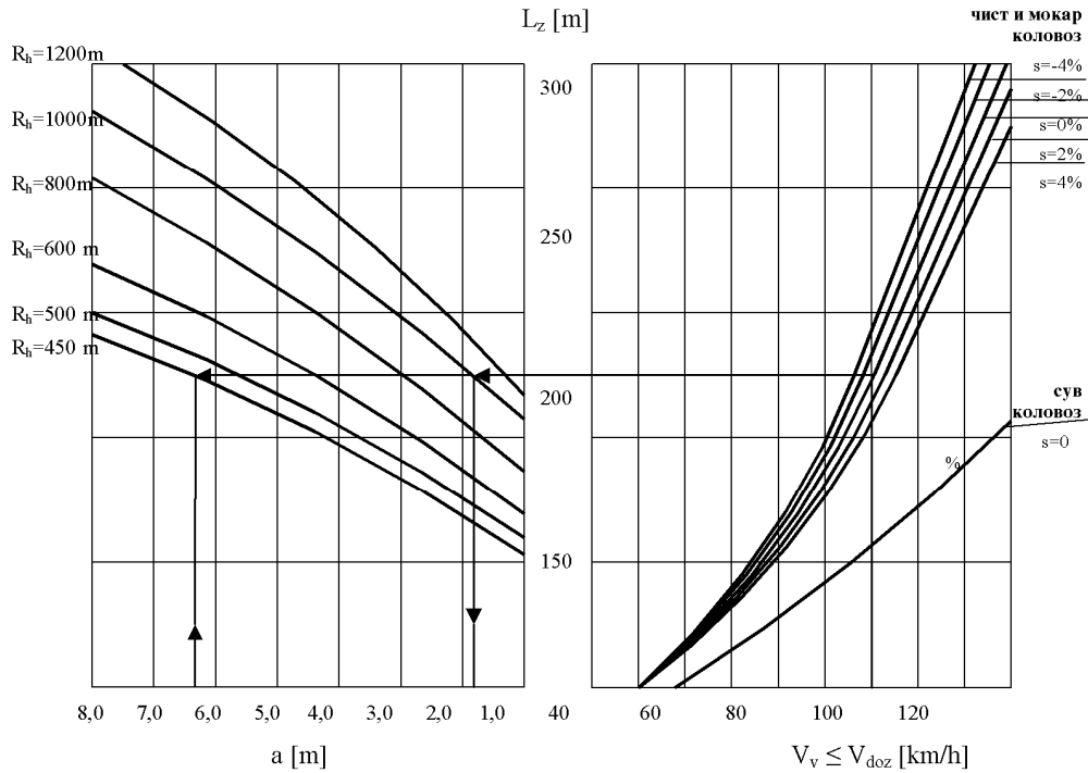
Слика 27. Меѓусебна зависност на радиусот R_h и оддалеченоста меѓу пречките и работ на крајната сообраќајна лента, а во функција од брзината V_v и од надолжниот наклон на нивелетата.
