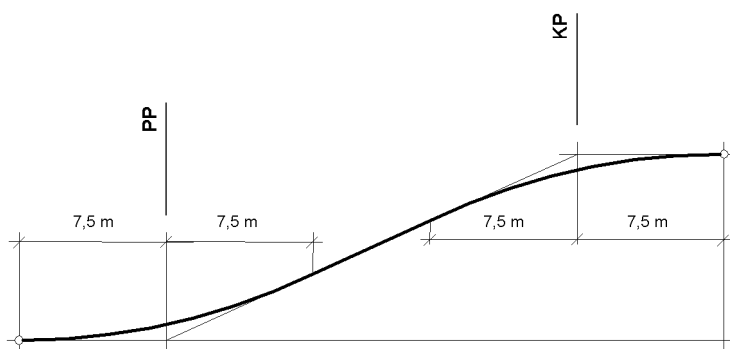
Слика 12. Проширување со заоблување
