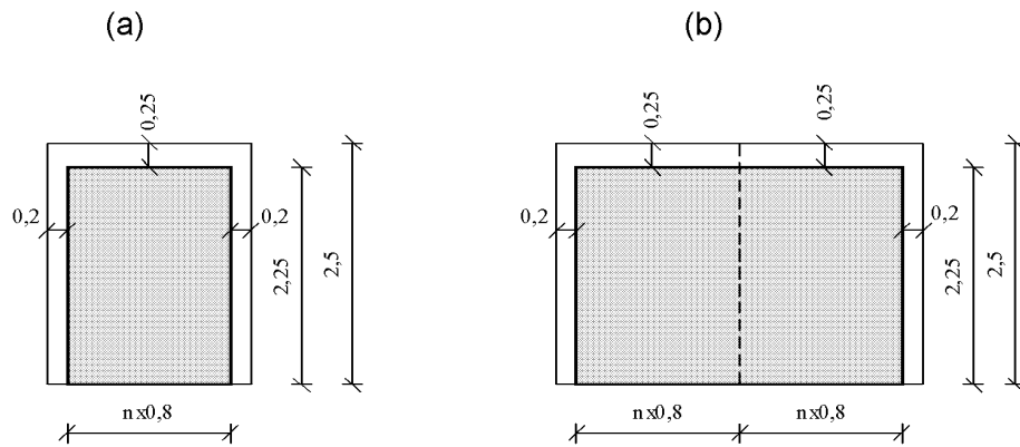
Слика 9. Сообраќаен и слободен профил на еднонасочна (а) и двонасочна (б) пешачка патека
